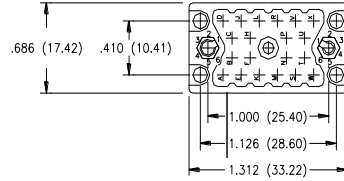
20 PIN RECEPTACLE
