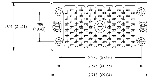
120 PIN RECEPTACLE
