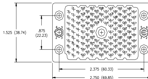
120 PIN RECEPTACLE
