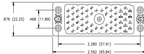
56 PIN RECEPTACLE
