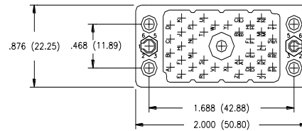
56 PIN RECEPTACLE
